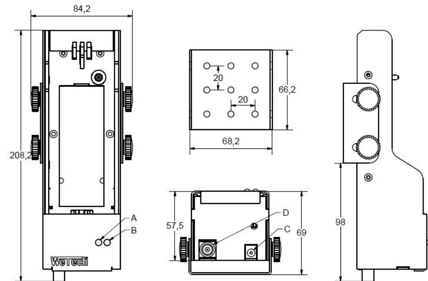
Schemazeichnung WTC623
